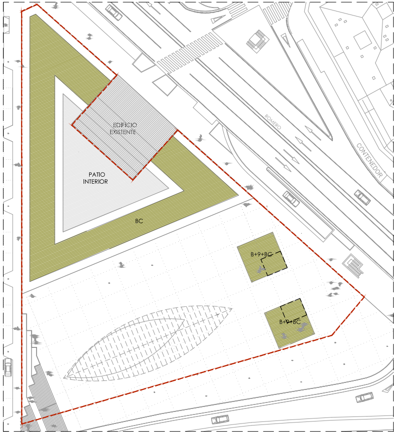
PLANTAS 7,8,9 -SUPERFICIE EDIFICADA POR PLANTA
