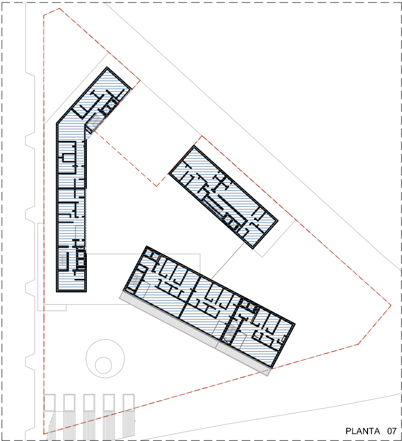
PLANTA 07
