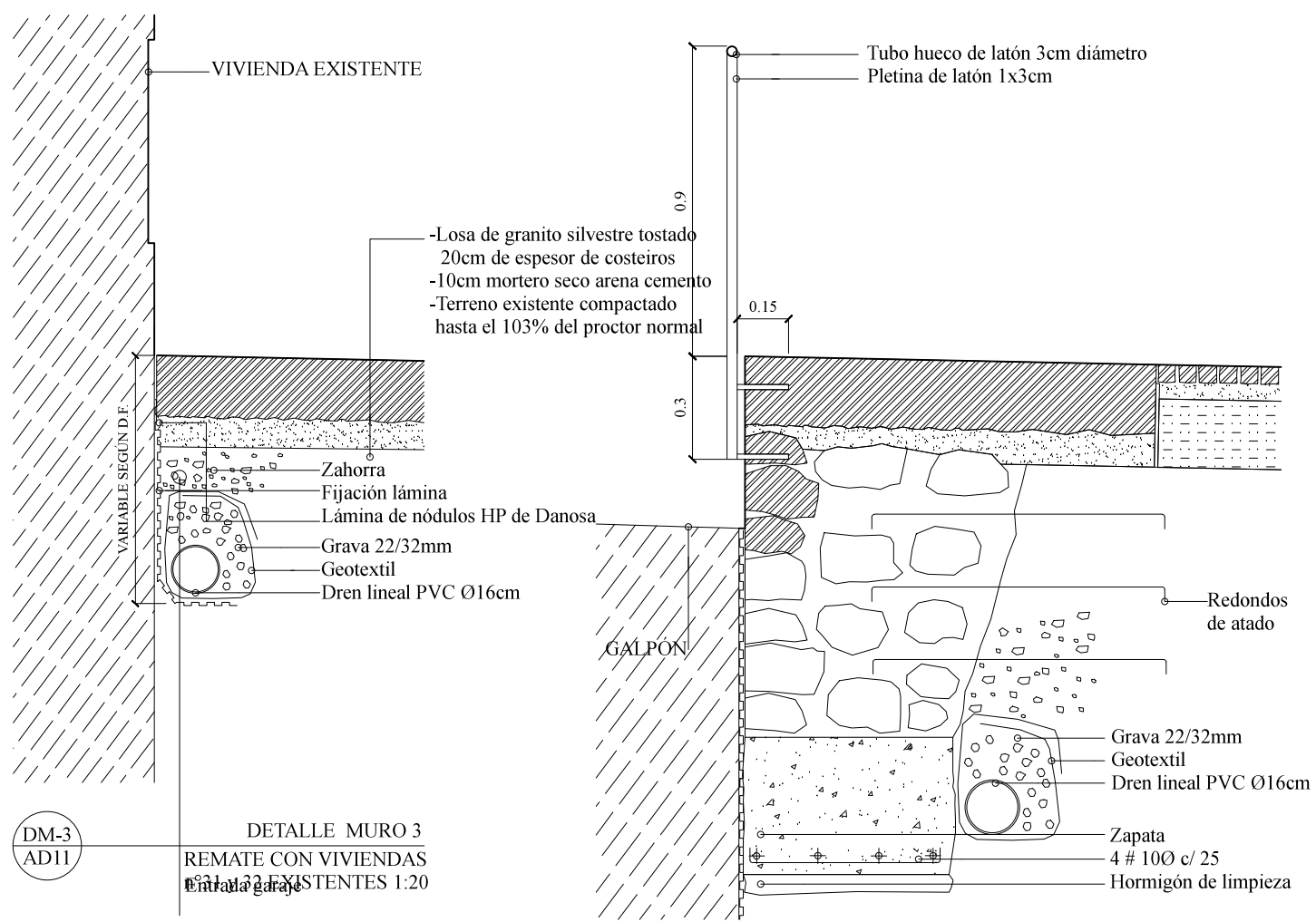
DM-4 AD11 DETALLE MURO 4 MURO REMATE CON GALPÓN VIENDA n° 32 1:20
