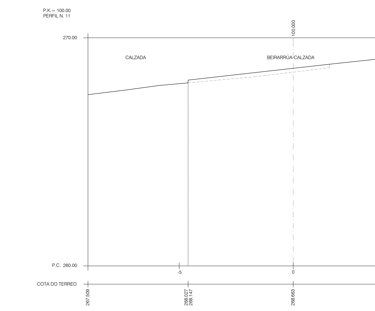
PERFIS TRANSVERSAIS E: 1/100
