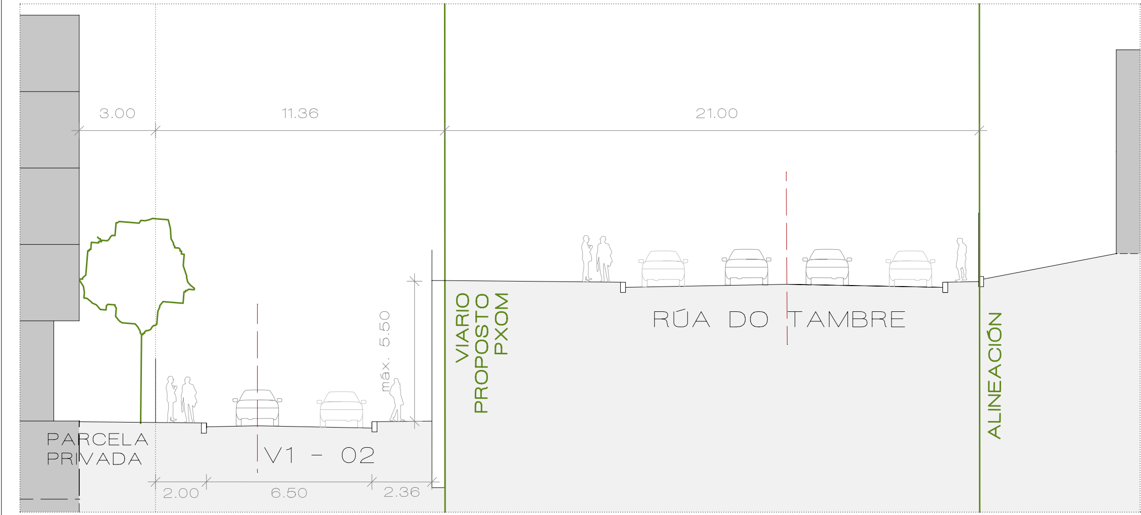
SECCIÓN B-B'
