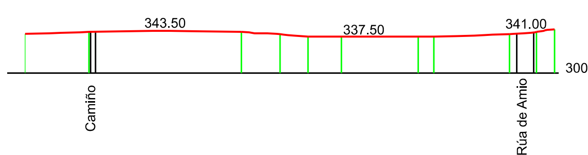
PERFIL C-C
