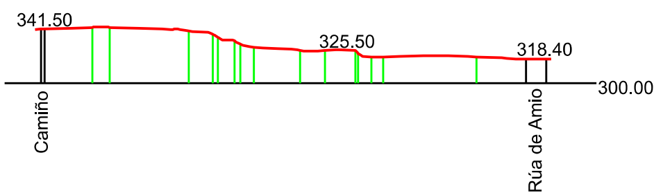
PERFIL B-B
