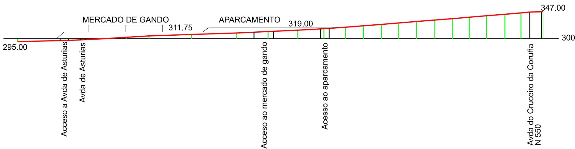
PERFIL B-B
