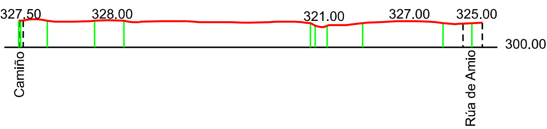
PERFIL E-E
