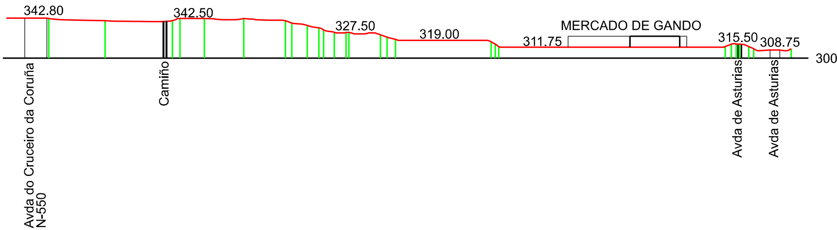
PERFIL D-D
